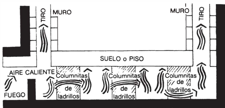
Plano de «hipocaustis»
