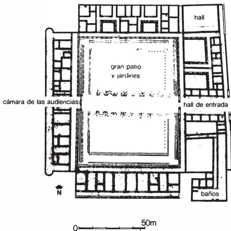
Planta del Palacio de Fishbourne
